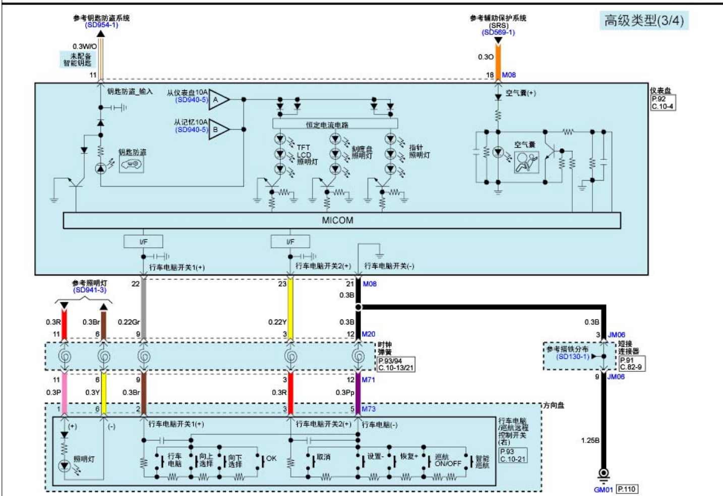
指示灯&amp;仪表(7)
